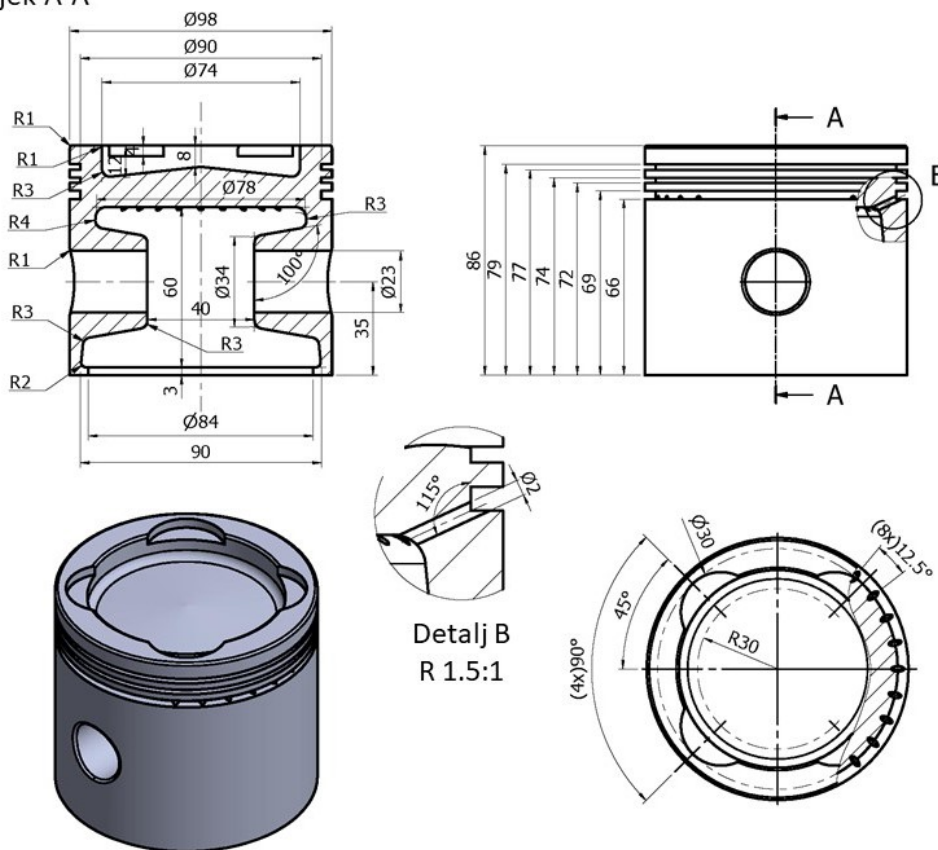
Presjek A-A
